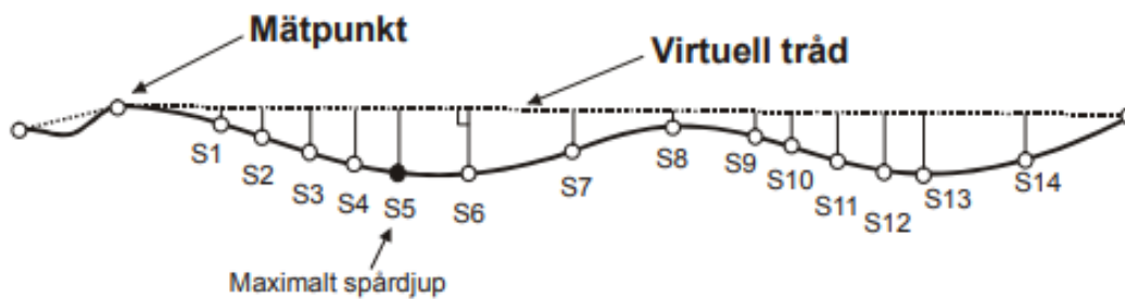
Figur 1: Beskrivning av trådprincipen för spårdjupsmätning. Figur hämtad från Vägytemätning Mätstorheter (TDOK 2014:0003) [27]
